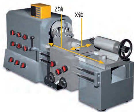
车床： 2轴 KA计数器 + 两个直线光栅尺
