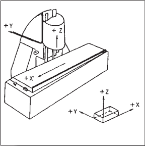
床式铣床
