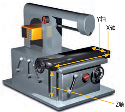
铣床： 3轴 KA计数器 + 三个直线光栅尺
