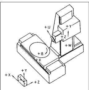
卧式镗床
