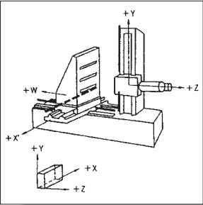
卧式镗铣床
