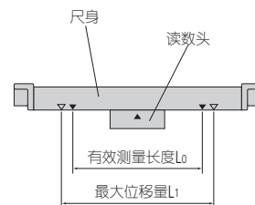
光栅尺
