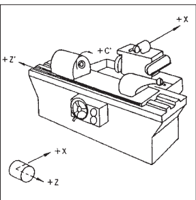
外圆磨床
