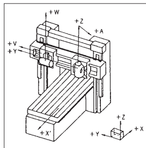
龙门铣床
