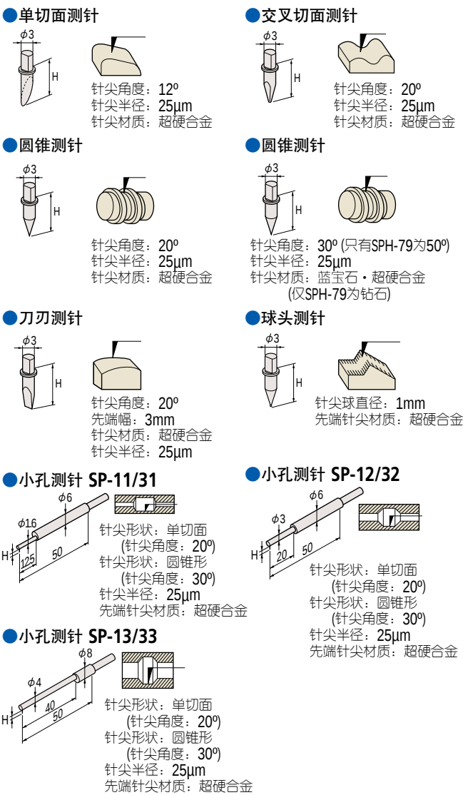
可应用测针列表(选件)
