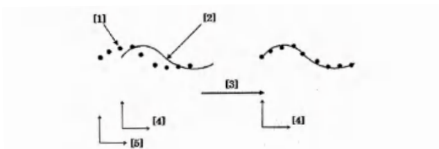
[1] 测量点 [2] 拟合数据参照文件 [3] 最佳拟合 [4] 标准坐标系 [5] 测量坐标系
