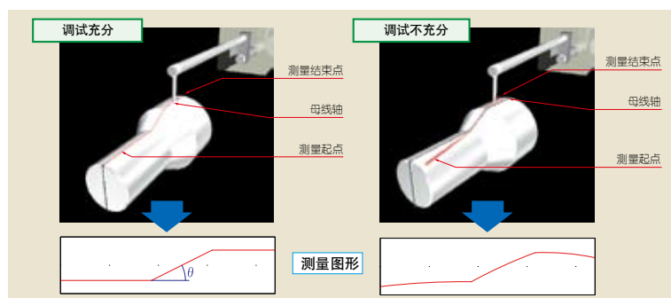
使用 3 轴调整工作台时的 FORMTRACEPAK 导向画面
